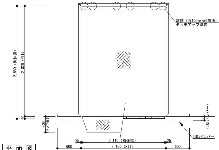
平面図
