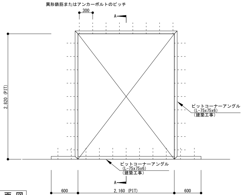
平面図
